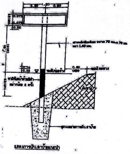
แสดงการปักเสาป้ายถนน
