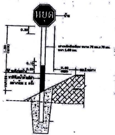
แสดงการปักเสาป้ายบังคับป้ายเตือน
